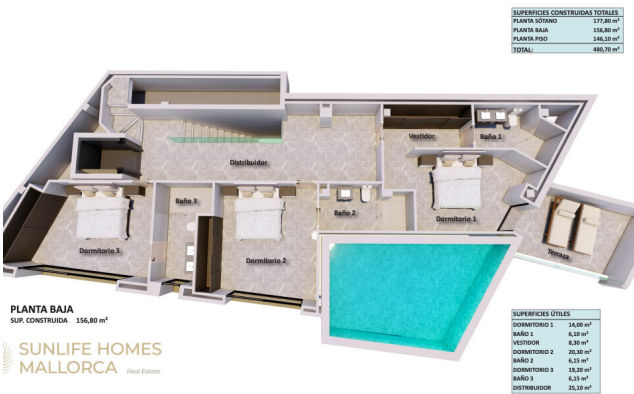
Plano - Nivel 2
